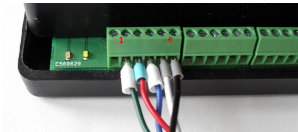
Abbildung 2: Anschlussbelegung Tür 1
